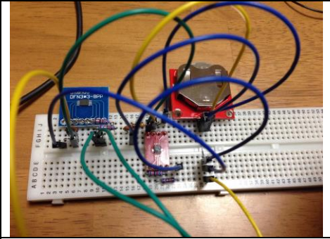
電池残量 IC 評価回路
